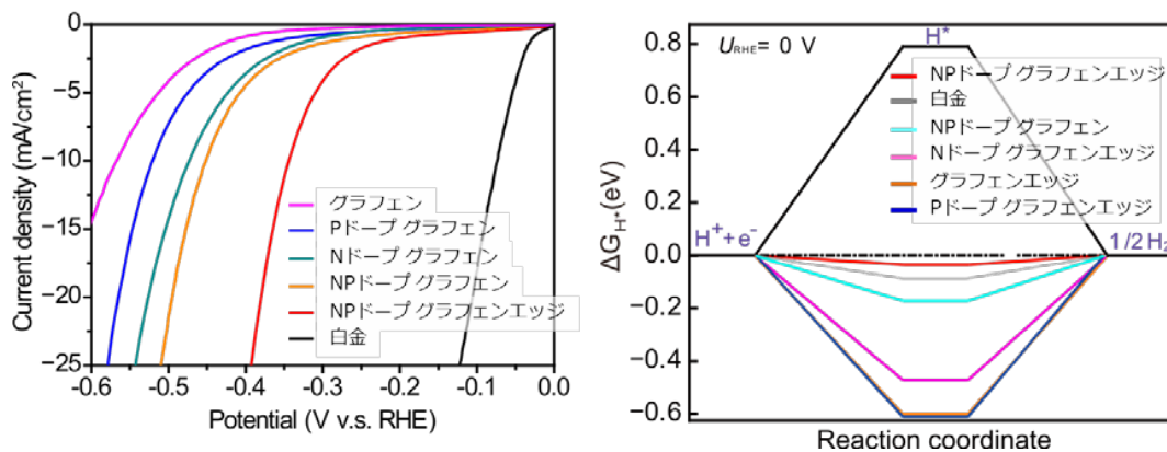
図 3 (左):ポテンシostatを用いた水素発生反応に関するサイクリックボルタンメトリー測定結果。電位を卑に掃引した場合の電流密度の変化を示しており、その反応開始電位と高い電流密度を得ることが、材料の水素が発生する反応性の高さを示す。グラフェンのエッジ構造に NP ドープを行った際に最も反応性が高いことが分かり、非金属のみで構成されているにもかかわらず、貴金属で一般的に用いられる白金に迫る特性が得られている。(右図):DFT 計算による各グラフェンと白金におけるプロトンの吸着エネルギー。NP ドープを行ったグラフェンエッジ構造が白金よりも抑制されており、高い電極触媒能が期待される。
