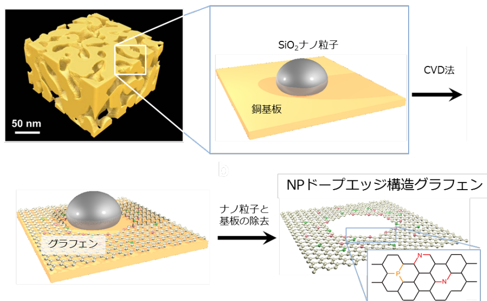
図 1 化学ドーブグラフェンエッジ構造の作製法の概略図。銅基板上に SiO 2 のナノ粒子を分散させ、CVD 法によりグラフェンを成長させる。グラフェンは、ナノ粒子上では成長せず、その後、ナノ粒子と基板を除去することでグラフェンにナノ粒子の粒径の大きさが開いたグラフェンエッジを作製し、CVD 法の導入ガスや成長温度を調整することで NP の化学ドーブを行った。導入された NP は挿入図の化学構造を持つピエリジン型を主に有する。
