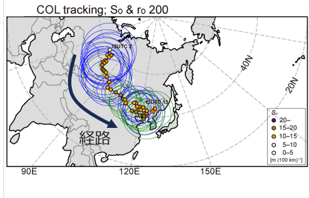
図2：（左図）大雨期間で平均した寒冷渦指標における等圧面の凹み具合。200hPaと500hPaをそれぞれ陰影と等値線で示している。（右図）最大降水量を記録した8/13に朝鮮半島付近に位置していた寒冷渦の移動経路。点は寒冷渦/トラフの位置、点の色はその強度、青/緑の円は渦の半径を示しそれぞれトラフ/寒冷渦に対応する。どちらも原著図に加筆。
